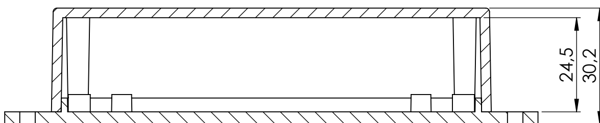
PRZEKRÓJ A-A
