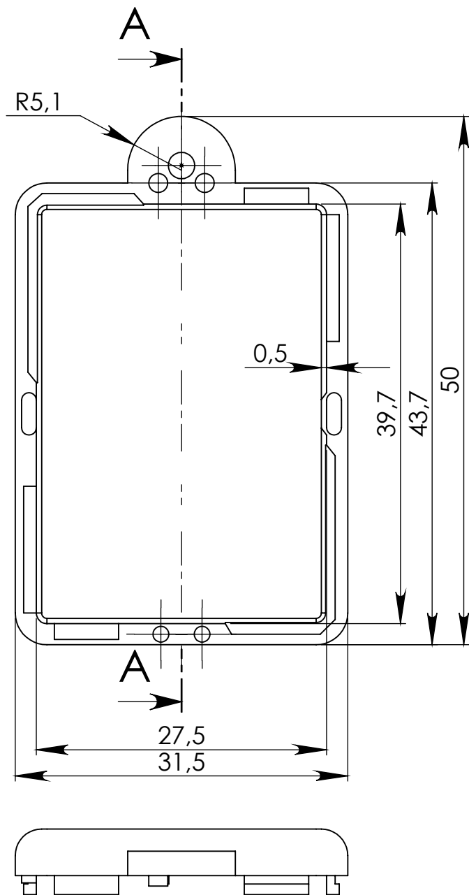
PRZEKRÓJ A-A SKALA 2 : 1
