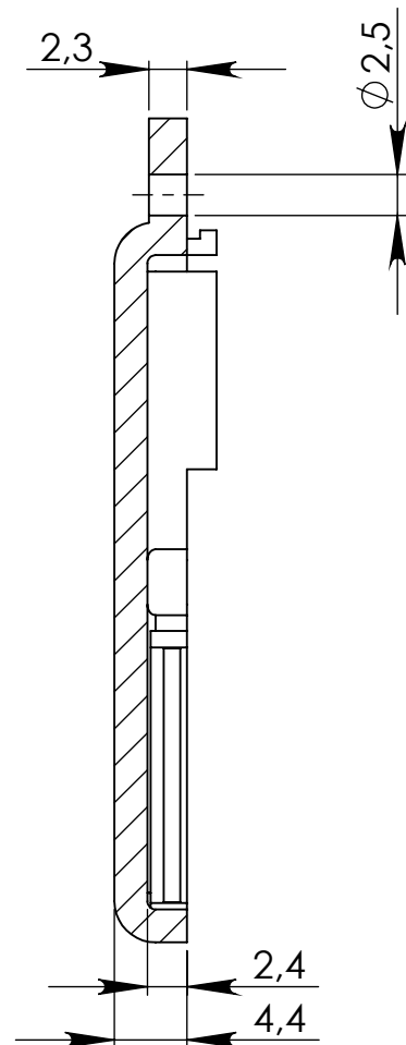
PRZEKRÓJ A-A SKALA 2 : 1
