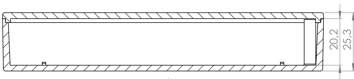
PRZEKRÓJ A-A
