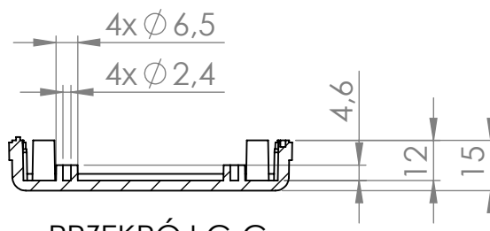
PRZEKRÓJ C-C
