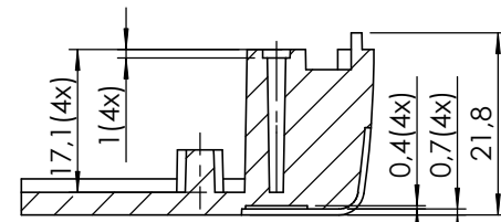
PRZEKRÓJ A-A SKALA 1 : 1
