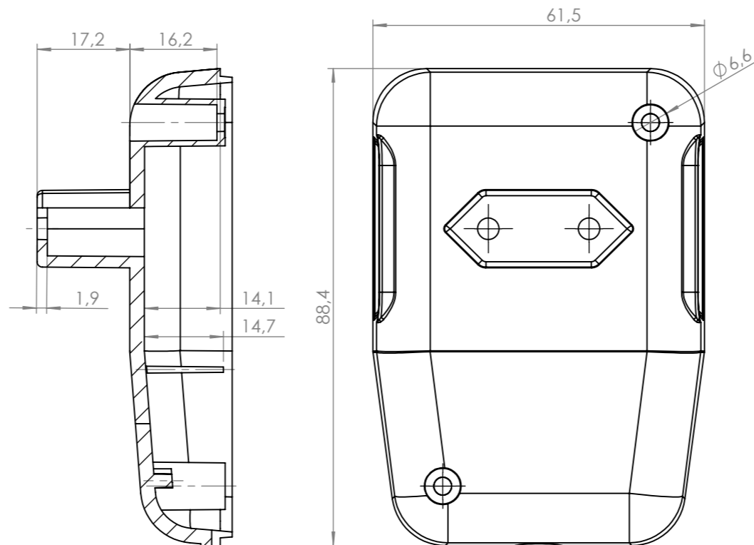
PRZEKRÓJ C-C SKALA 1 : 1
