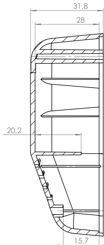
PRZEKRÓJ A-A SKALA 1 : 1
