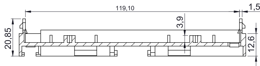
PRZEKRÓJ A-A
