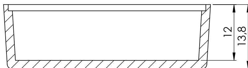
PRZEKRÓJ B-B
