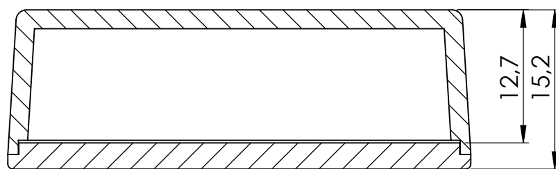
PRZEKRÓJ A-A
